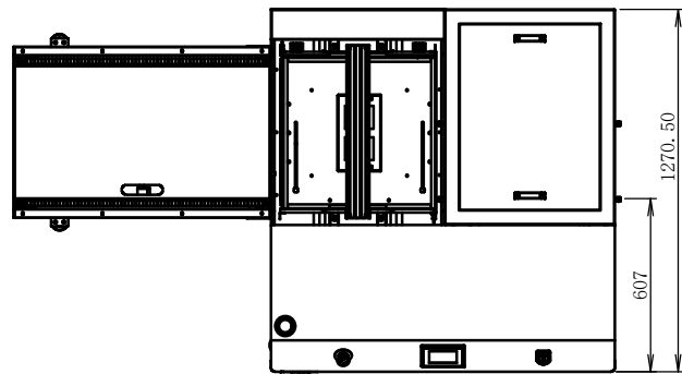
标准XL号吸送一体机（左到右）
