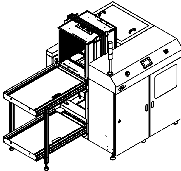
标准XL号吸送一体机（左到右）
