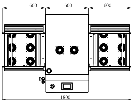
XL-600-缓存机 (双丝杆) (双边带0.6米轨道)
